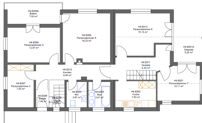
1. Obergeschoss Haus K
