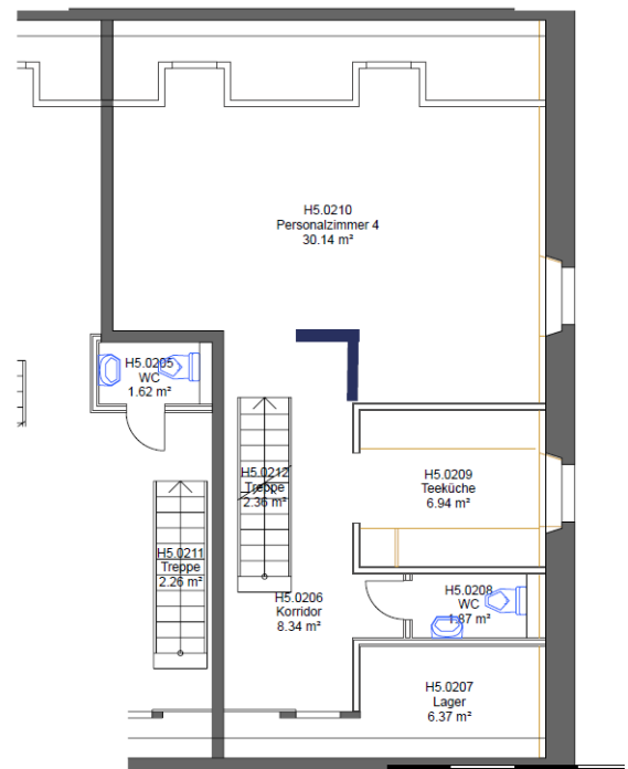
2. Obergeschoss Haus F
