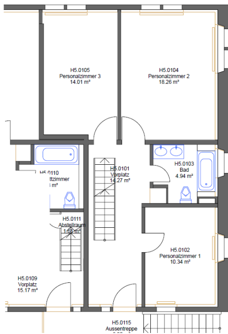
1. Obergeschoss Haus F
